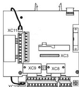
Figura 2: Encaje del conector XC11 - EBA/EBB - Vista superior
