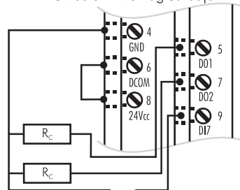
Figura 8: Configuración de las entradas y salidas digitales para ACTIVO en nivel lógico BAJO
