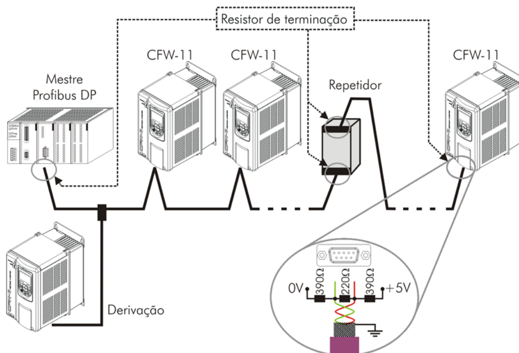
Figura 2.1 – CFW-11 em rede Profibus DP
