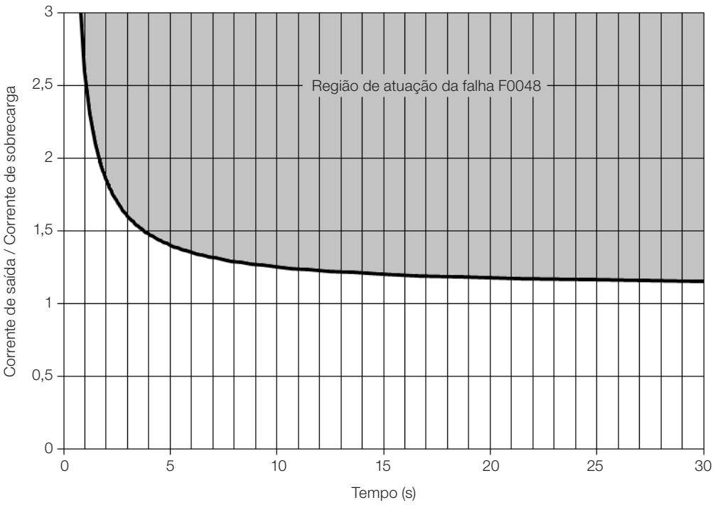
Figura 17.3: Atuação da sobrecarga dos IGBTs (Normal Duty - ND)
