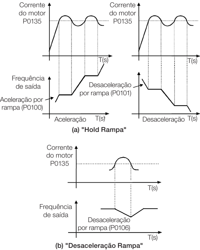
Figura 9.10: (a) e (b) Modos de atuação da Limitação de Corrente via P0135
