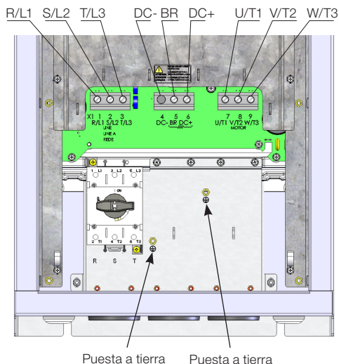
(d) Tamaño D con grado de protección IP55
