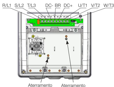
(b) Mecânicas B e C com grau de proteção IP55
