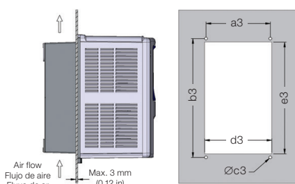
(b) Flange mounting (b) Montaje en flange (b) Montagem em flange
