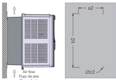
(a) Surface mounting (a) Montaje en superficie (a) Montagem em superfície
