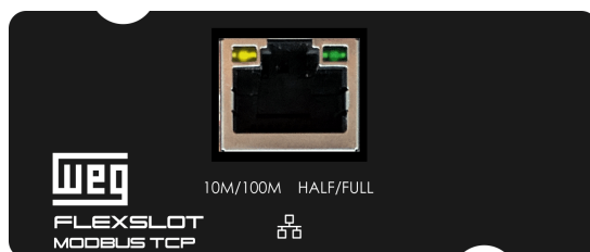
Figura 3.10: Modbus TCP
