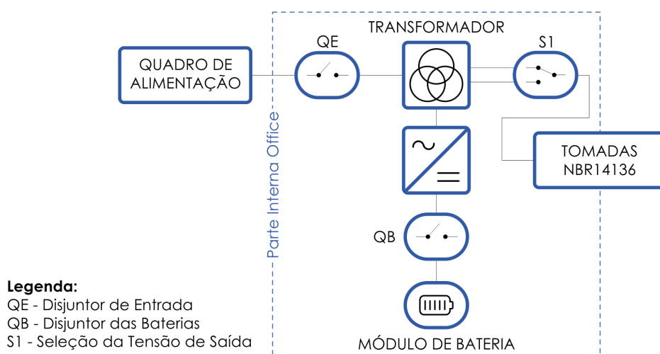
Figura 5.3: Modelo com baterias internas
