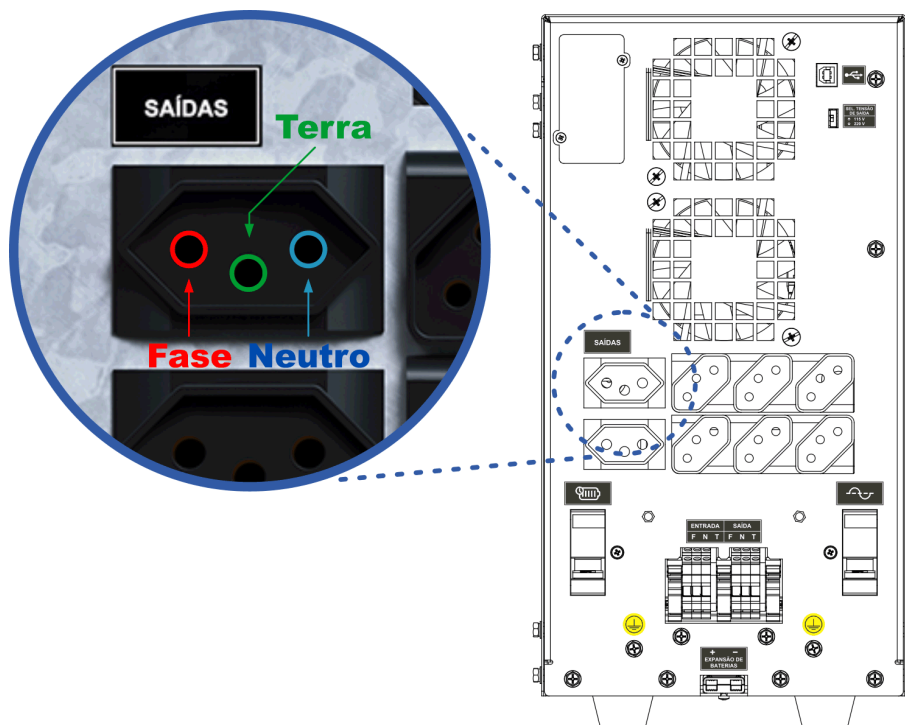
Figura 5.6: Polarização das tomadas de saída
