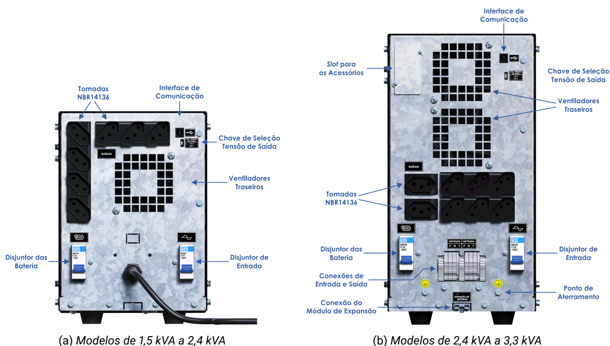
Figura 3.7: Detalhes do painel traseiro do Office Senoidal
