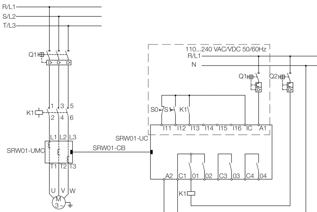
Figura 5.4: Esquema de ligação para o modo de operação Partida Direta utilizando entradas digitais em 24 Vcc e acionamento por botoeiras (P230 = 1)
