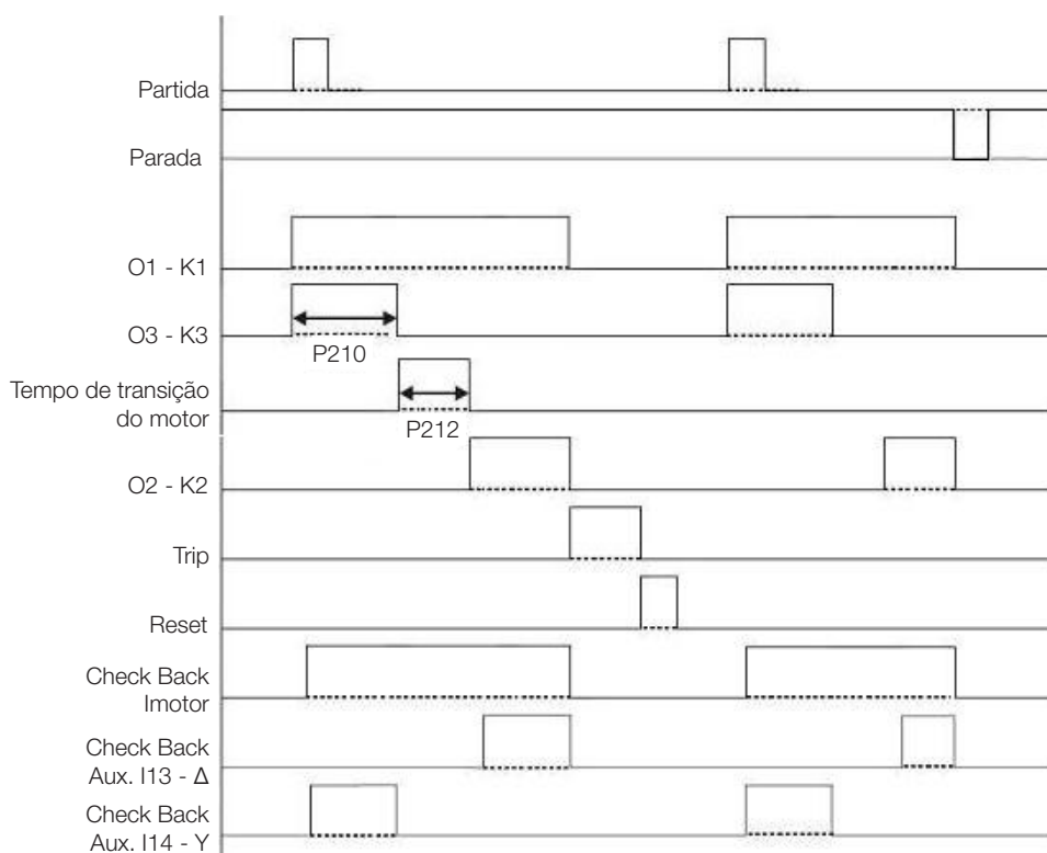
Figura 5.12: Diagrama de funcionamento para o modo de operação Partida Estrela-Triângulo
