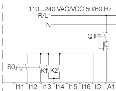
Figura 5.17: Detalhe modificação para acionamento utilizando entradas digitais em 24 Vcc e acionamento por chave ( P230 = 0 )
