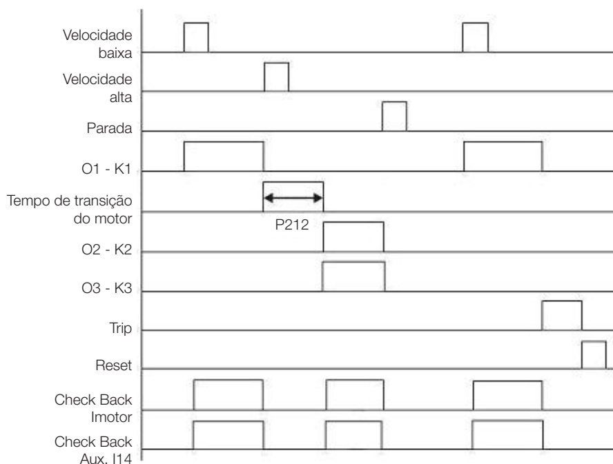
Figura 5.15: Diagrama de funcionamento para o modo de operação Partida Dahlander
