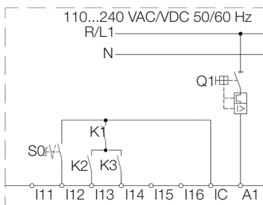
Figura 5.11: Detalhe modificação para acionamento utilizando entradas digitais em 24 Vcc e acionamento por chave (P230 = 0)
