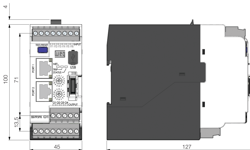
Figura 8.2: Dimensões da Unidade de Controle – UC (mm)
