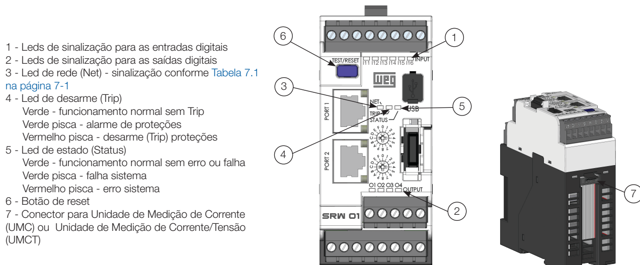
Figura 2.1: Identificação da Unidade de Controle do SRW 01
