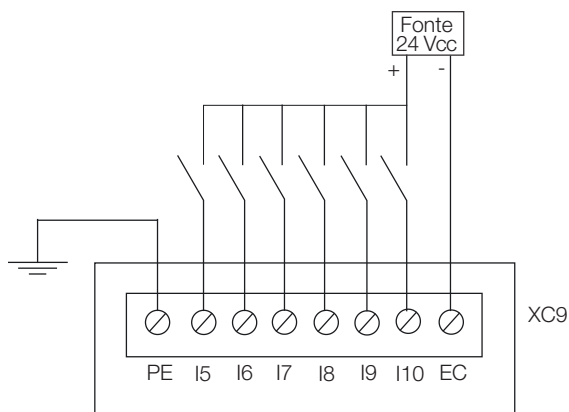
Figura 3.9: Acionamento das entradas digitais 24 Vcc
