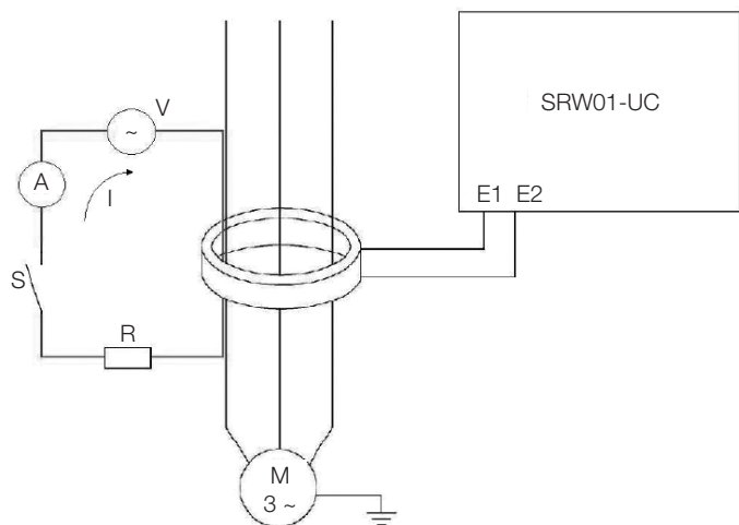
Figura 5.21: Esquema ligação para teste do circuito de medição da corrente de fuga à terra
