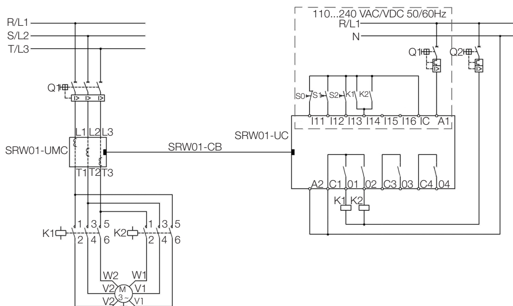
Figura 5.16: Esquema de ligação para o modo de operação Partida Dois Enrolamentos utilizando entradas digitais em 24 Vcc e acionamento por botoeiras ( P230 = 1 )
