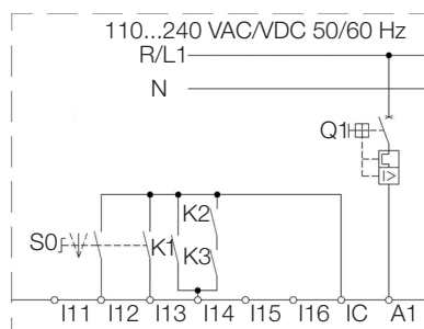
Figura 5.14: Detalhe modificação para acionamento utilizando entradas digitais em 24 Vcc e acionamento por chave ( P230 = 0 )
