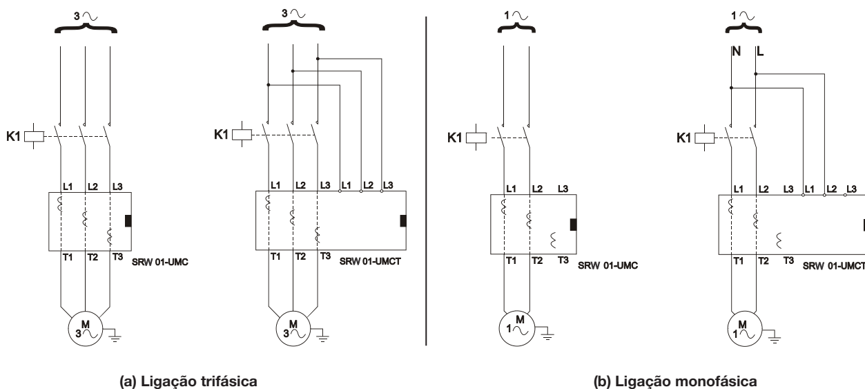
Figura 3.3: (a) e (b) Ligação trifásica e monofásica da Unidade de Medição de Corrente (UMC) e Unidade de Medição de Corrente/Tensão (UMCT)
