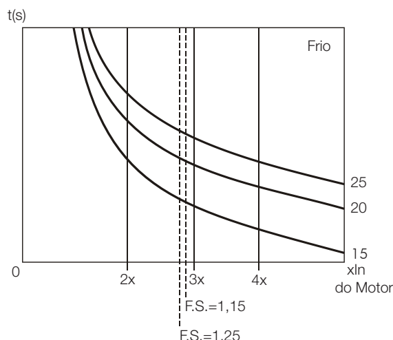
Figura 5.25: Utilizando o F.S. para identificar o novo tempo
