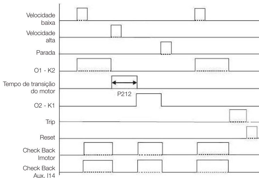
Figura 5.18: Diagrama de funcionamento para o modo de operação Partida Dois Enrolamentos
