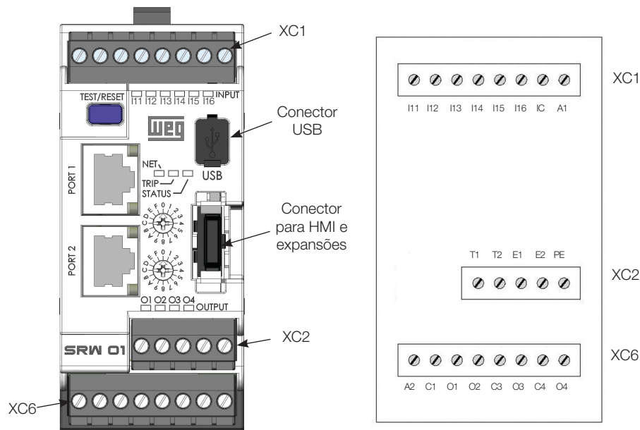
Figura 3.2: Conexões da Unidade de Controle
