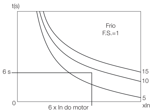
Figura 5.27: Verificando a classe mínima nas curvas a frio
