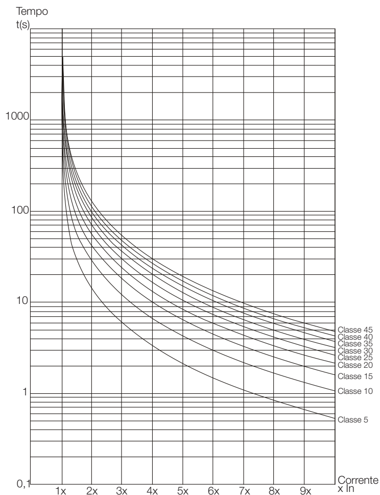
Figura 5.24: Classes de disparo para proteção do motor a quente com 100 % In
