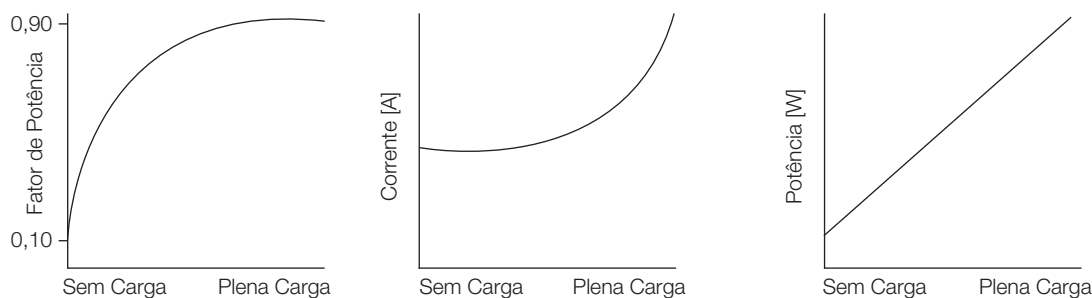
Figura 5.29: Comportamento do fator de potência, corrente e potência em razão da carga aplicada
