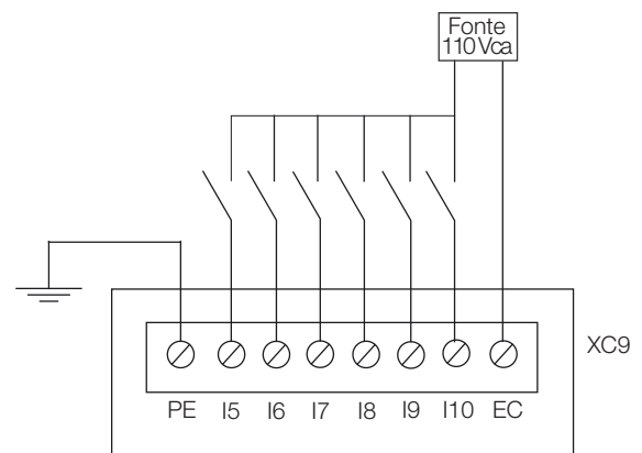
Figura 3.10: Acionamento das entradas digitais 110 Vca
