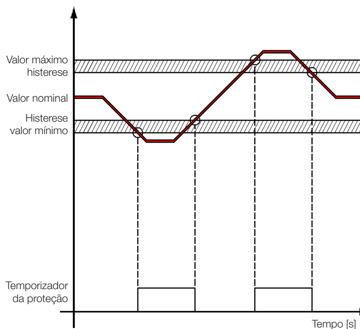
Figura 5.20: Aplicação de histerese
