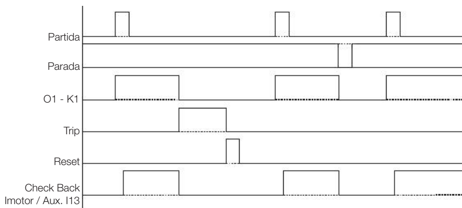
Figura 5.6: Diagrama de funcionamento para o modo de operação Partida Direta
