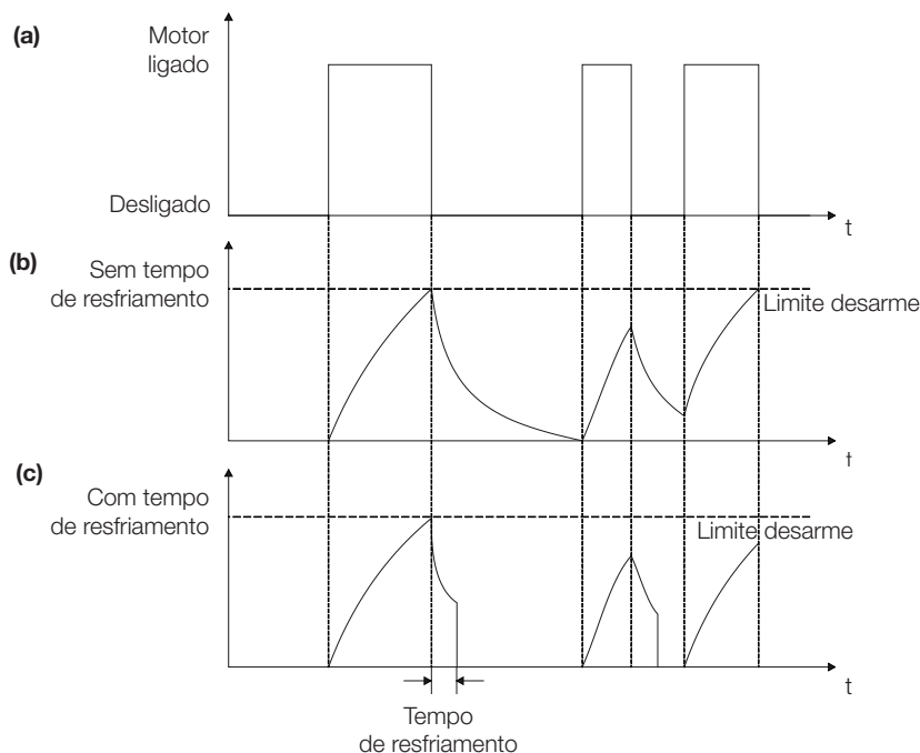
Figura 5.26: (a) a (c) Proteção de sobrecarga com e sem tempo de resfriamento
