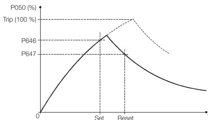
Figura 5.22: Programação do pré-alarme da proteção por sobrecarga
