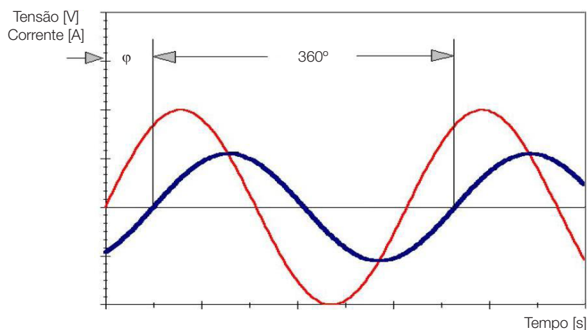
Figura 2.5: Defasagem entre os sinais de tensão e corrente
