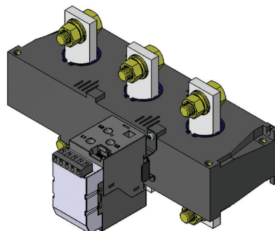
(l) Unidade de Medição de Corrente/Tensão - SRW 01-UMCT 6 (840 A/690 V) - com acessório barramento
