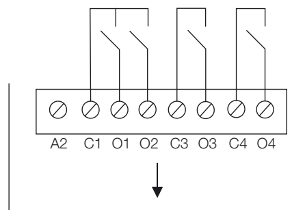
Figura 3.8: Esquema de ligação às saídas digitais
