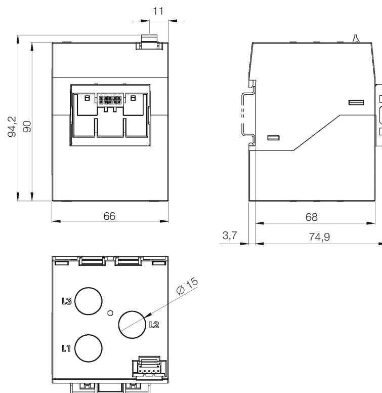
Figura 8.4: Dimensões da Unidade de Medição de Corrente – UMC 4 (mm)
