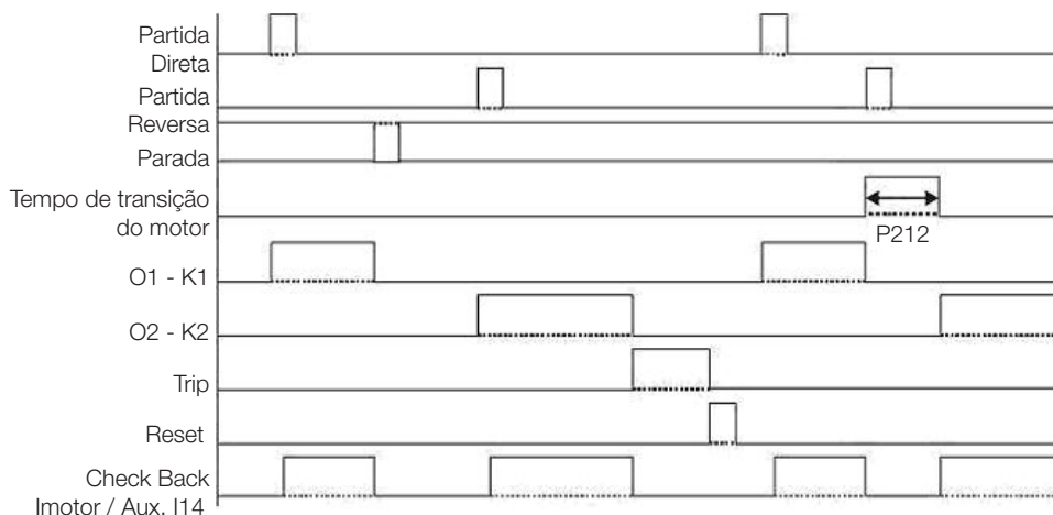
Figura 5.9: Diagrama de funcionamento para o modo de operação Partida Reversora
