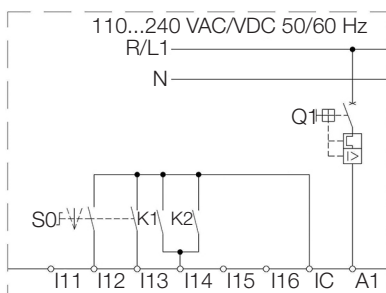
Figura 5.8: Detalhe modificação para acionamento utilizando entradas digitais em 24 Vcc e acionamento por chave (P230 = 0)
