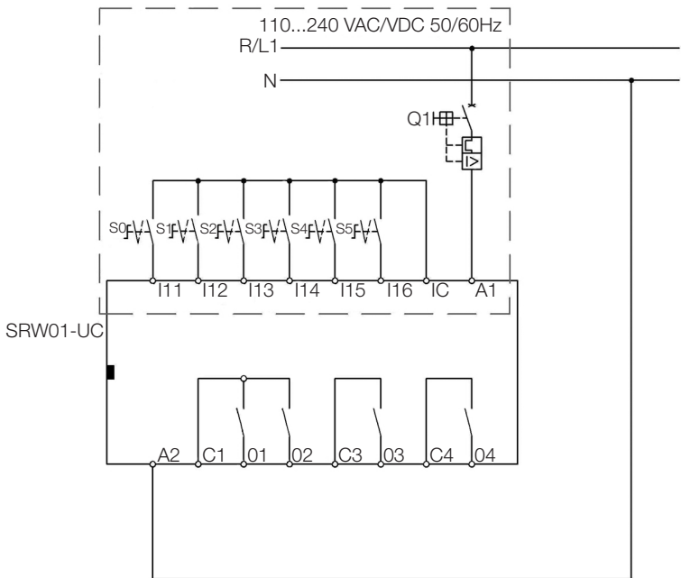
Figura 5.19: Esquema de ligação para o modo de operação PLC utilizando entradas digitais em 24 Vcc
