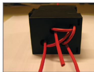
Figura 3.4: Conexão para faixa de corrente de 0,25 - 2,5 A - duas espiras na UMC1
