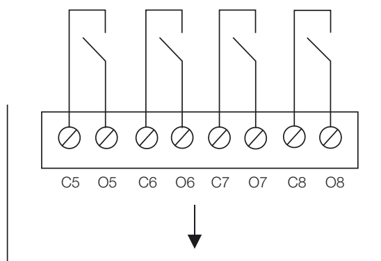
Figura 3.11: Esquema de ligação às saídas digitais
