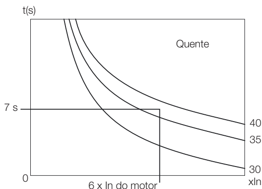
Figura 5.28: Verificando a classe de disparo máxima nas curvas a quente
