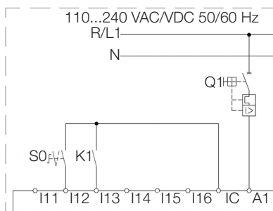
Figura 5.5: Detalhe da modificação para acionamento utilizando entradas digitais em 24 Vcc e acionamento por chave (P230 = 0)
