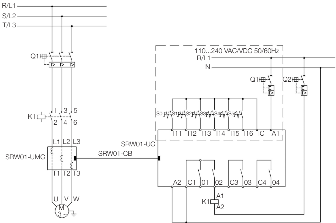
Figura 5.3: Esquema de ligação para o modo de operação Relé de Sobrecarga utilizando entradas digitais em 24 Vcc
