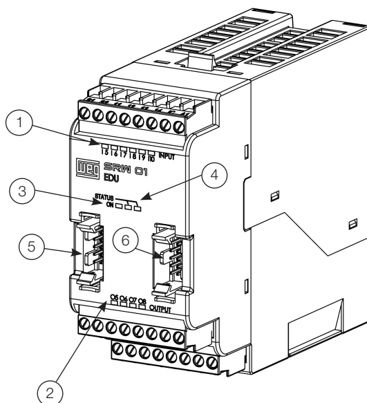
(n) Unidade de Expansão Digital – SRW 01-EDU
