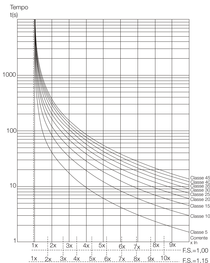
Figura 5.23: Classes de disparo para proteção do motor a frio
