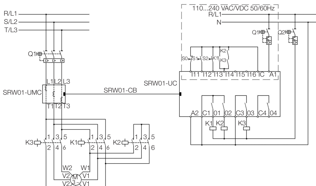
Figura 5.13: Esquema de ligação para o modo de operação Partida Dahlander utilizando entradas digitais em 24 Vcc e acionamento por botoeiras ( P230 = 1 )
