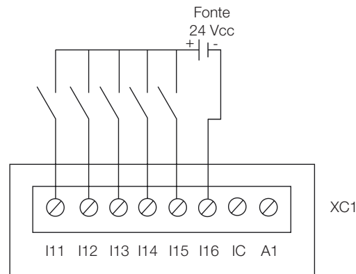
Figura 3.7: Conexão de fonte 24 Vcc externa
