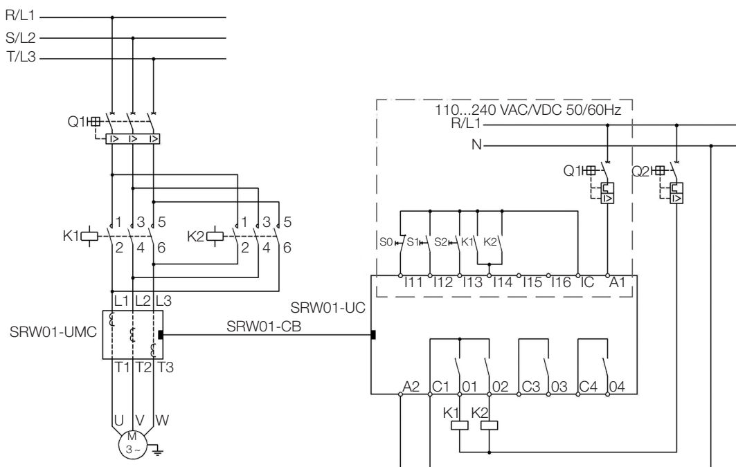
Figura 5.7: Esquema de ligação para o modo de operação Partida Reversora utilizando entradas digitais em 24 Vcc e acionamento por botoeiras (P230 = 1)
