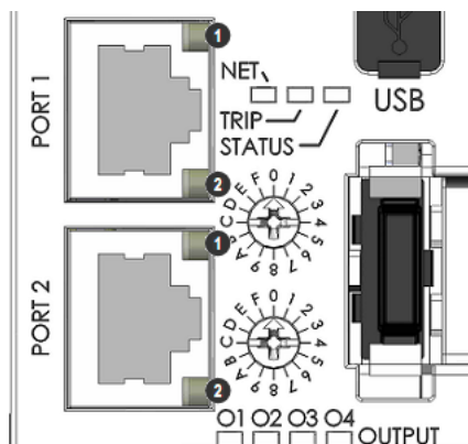
Figura 3.1: Conectores e LEDs
