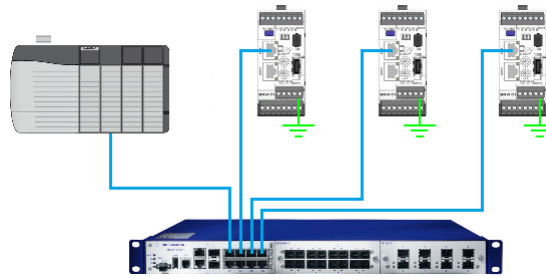
Figura 4.1: Topologia estrela
